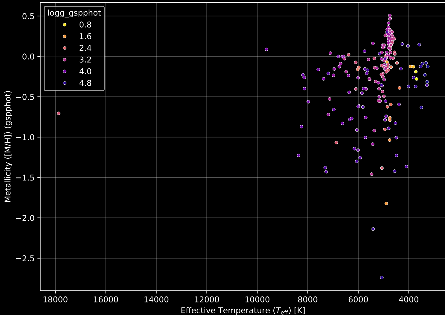
APOGEE DR17 Field: [K2_C11_005+07_btx] Stellar Population Parameters (n= 193)
